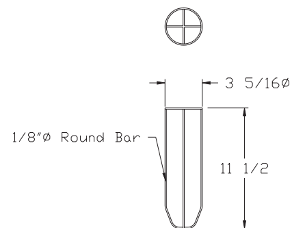
BACKFLUSH RESTRAINER
